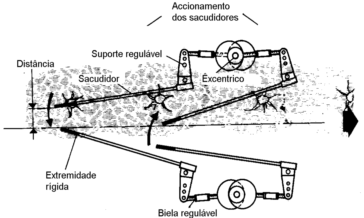
Representação de um conjunto de batedores direitos
