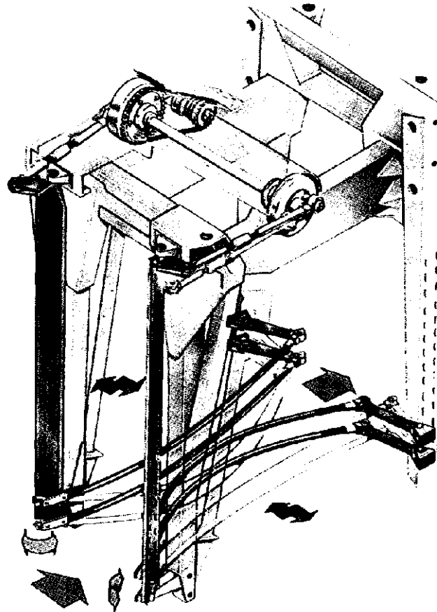
Representação do sistema de vibradores SDC
