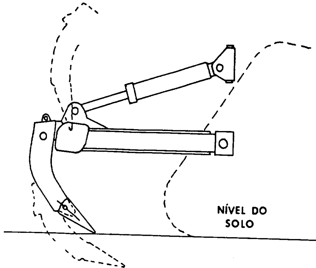
Representação de um “ripper” radial com um dente
