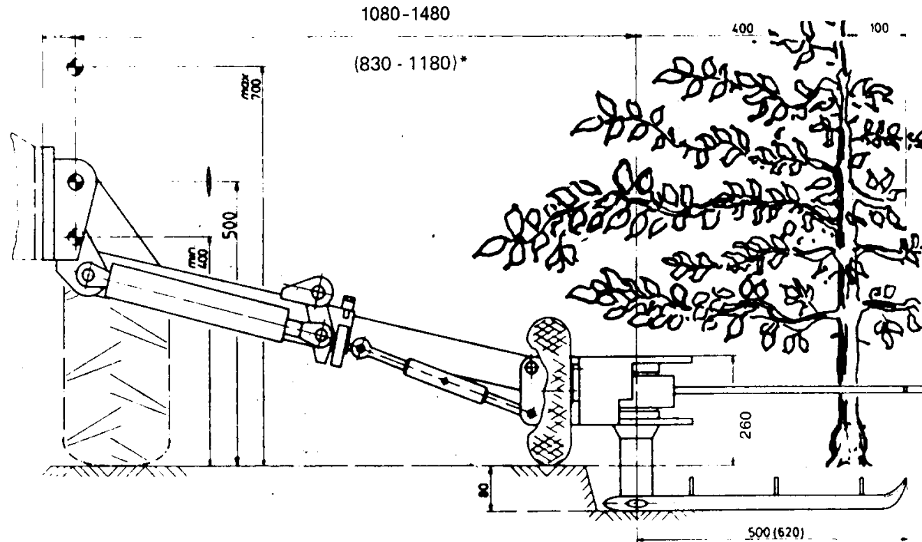
Representação de um intercepas de facas
