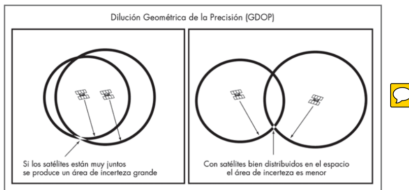
Figura 2.8: Influencia de la distribución de los satélites en el espacio sobre el nivel de precisión obtenido, GDOP.
