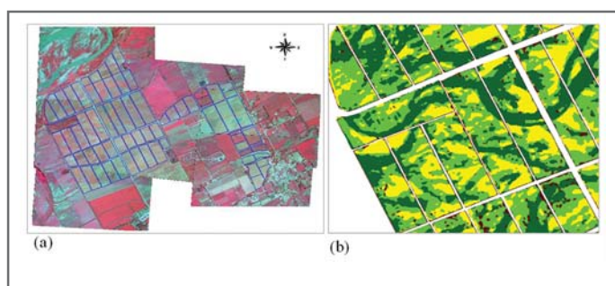
Figura 3.11: (a) Imagen multiespectral corregida de un viñedo y dispuestas en un mosaico. (b) Visualización de la clasificación de Índice vegetal NDVI.
