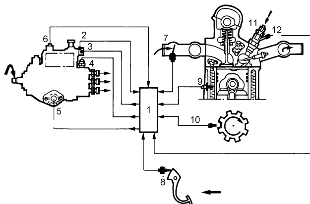
Figura 3- Princípio de funcionamento de um sistema de injeção com comando electrónico
