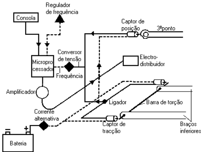
Figura 4- Representação geral do sistema hidráulico de elevação das alfaias com regulação electrónica Fonte: BP Nº 138 (1982)
