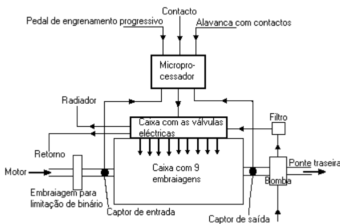
Figura 2- Exemplo de uma caixa de velocidades de comando electrónico Fonte: BP Nº 156 (1991)
