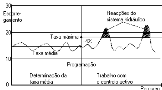
Figura 1 - Programação da taxa máxima de escorregamento em função da taxa média Fonte: BP Nº 156 (1991)
